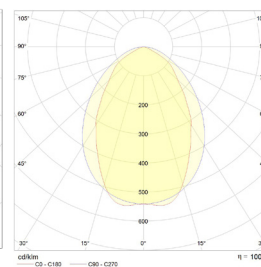
Tunneli keskileveä 60 (T60)
